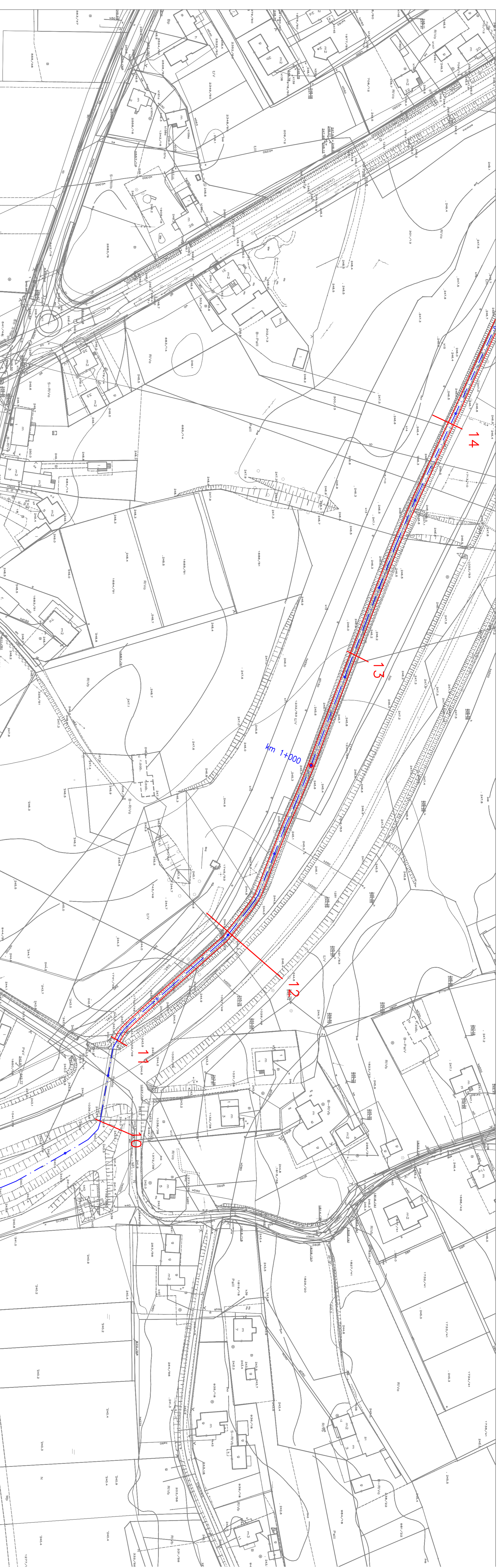
Rys. 3.5. Plan sytuacyjny cz. 5 Skala 1:1000
